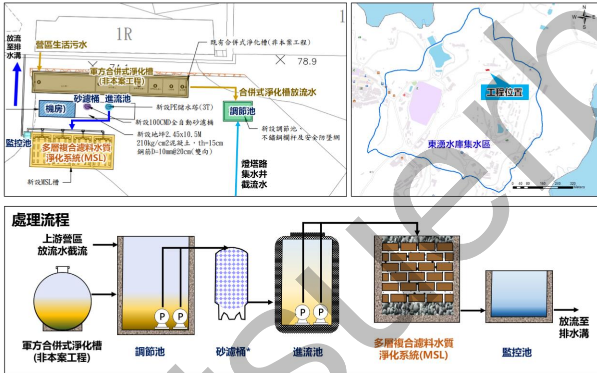
圖 4 東湧水庫集水區水質淨化設施工程內容示意圖
